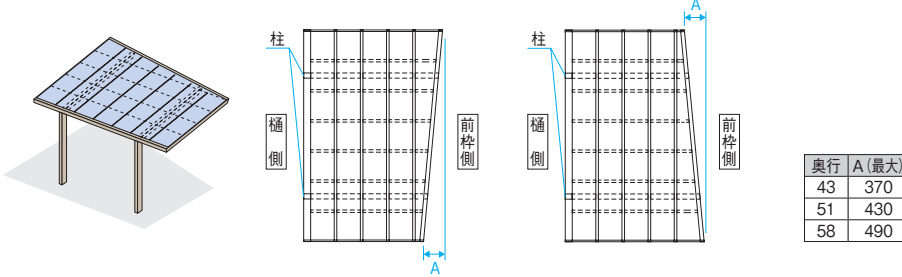
隅切り納まり/アーバングレー/基本タイプ/4327/H22/ポリカーボネート板: ブレースモーク ※間口33は柱3本になります。
