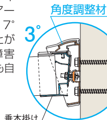
垂木掛け
