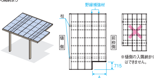
隅切り納まり / アーバングレー / 基本タイプ / 4327 (2200mm) / ポリカーボネート板: ブレースマーク ※間口33は柱3本になります。
